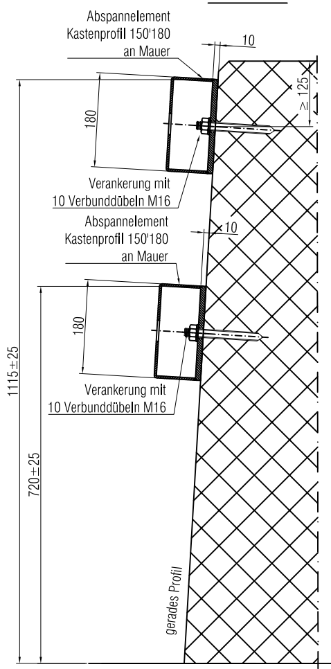
Schnitt A-A
