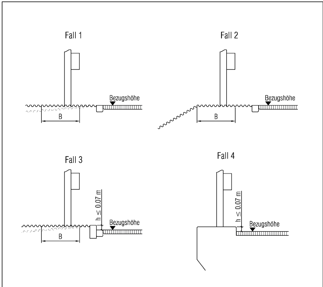
Abb. 6.1 Positionen und Bezugshöhen System 6211 (Anwendung, siehe Ziffer 6.2).
