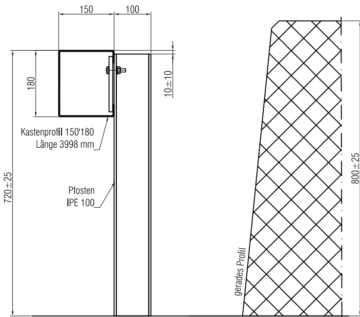
Schnitt B-B
