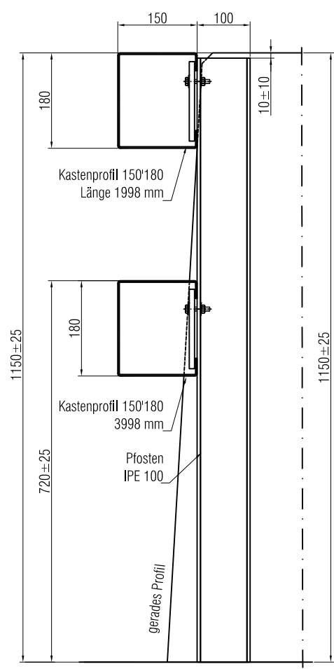
Schnitt B-B
