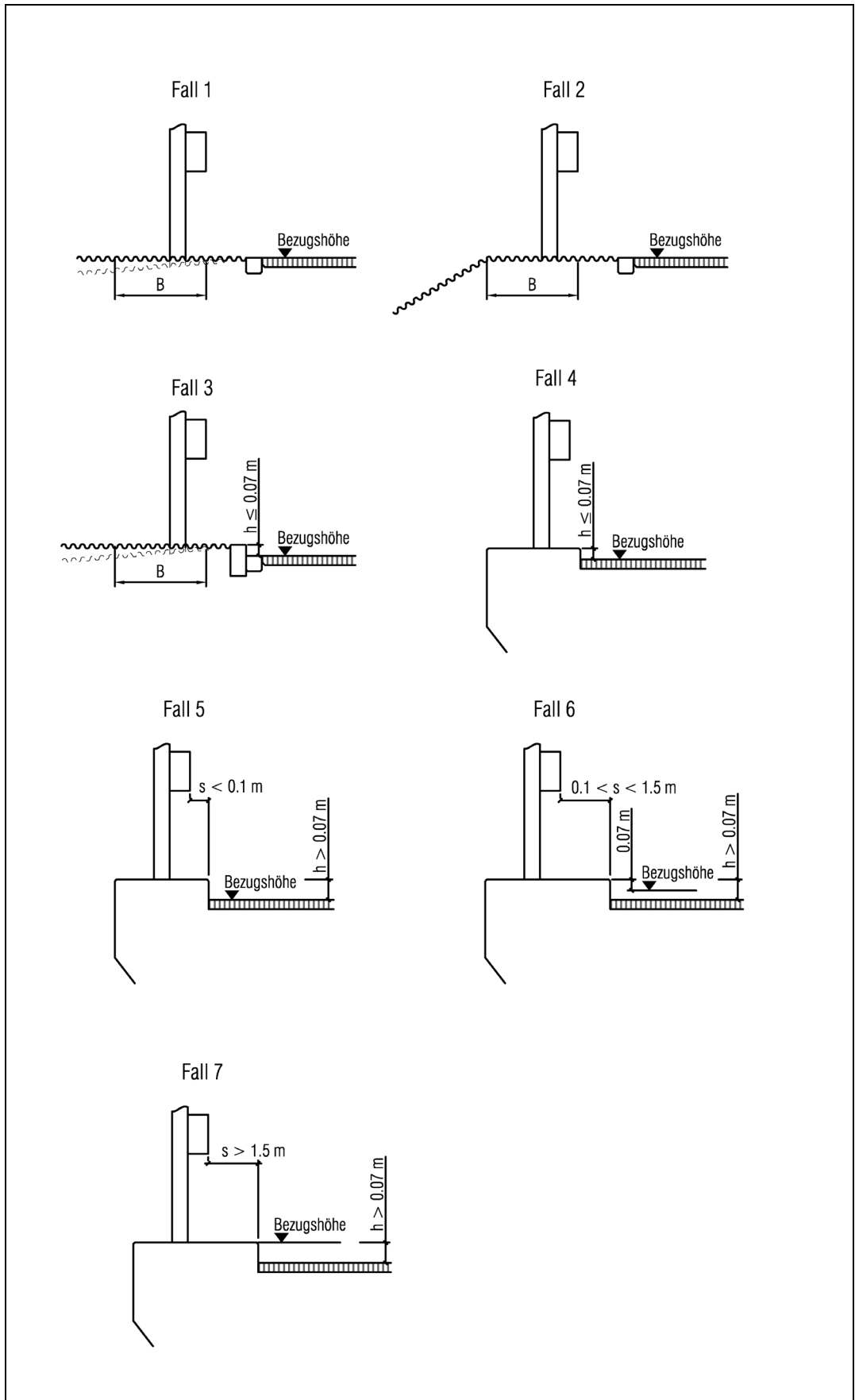
Abb. 6.1 Positionen und Bezugshöhen System 4311 (Anwendung, siehe Ziffer 6.2).
