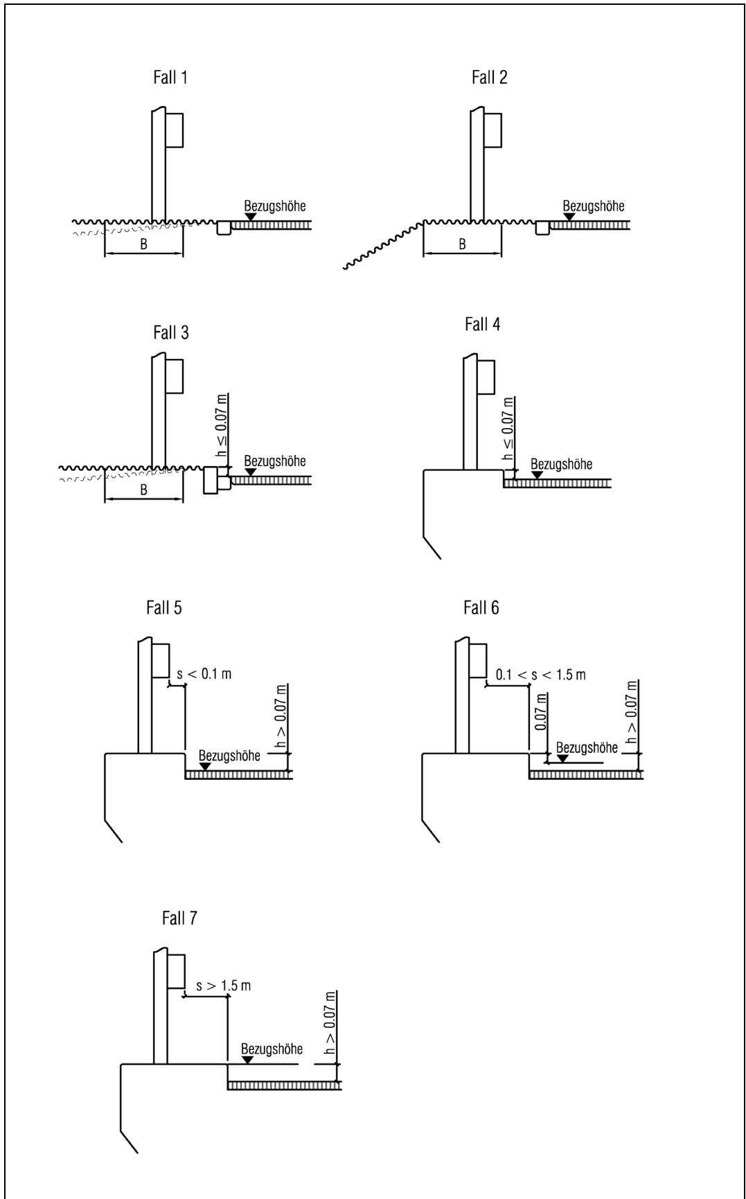
Abb. 6.1 Positionen und Bezugshöhen System 2211 (Anwendung, siehe Ziffer 6.2).
