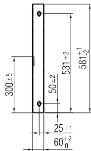
Ansicht von B
