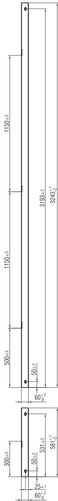
Ansicht von B
