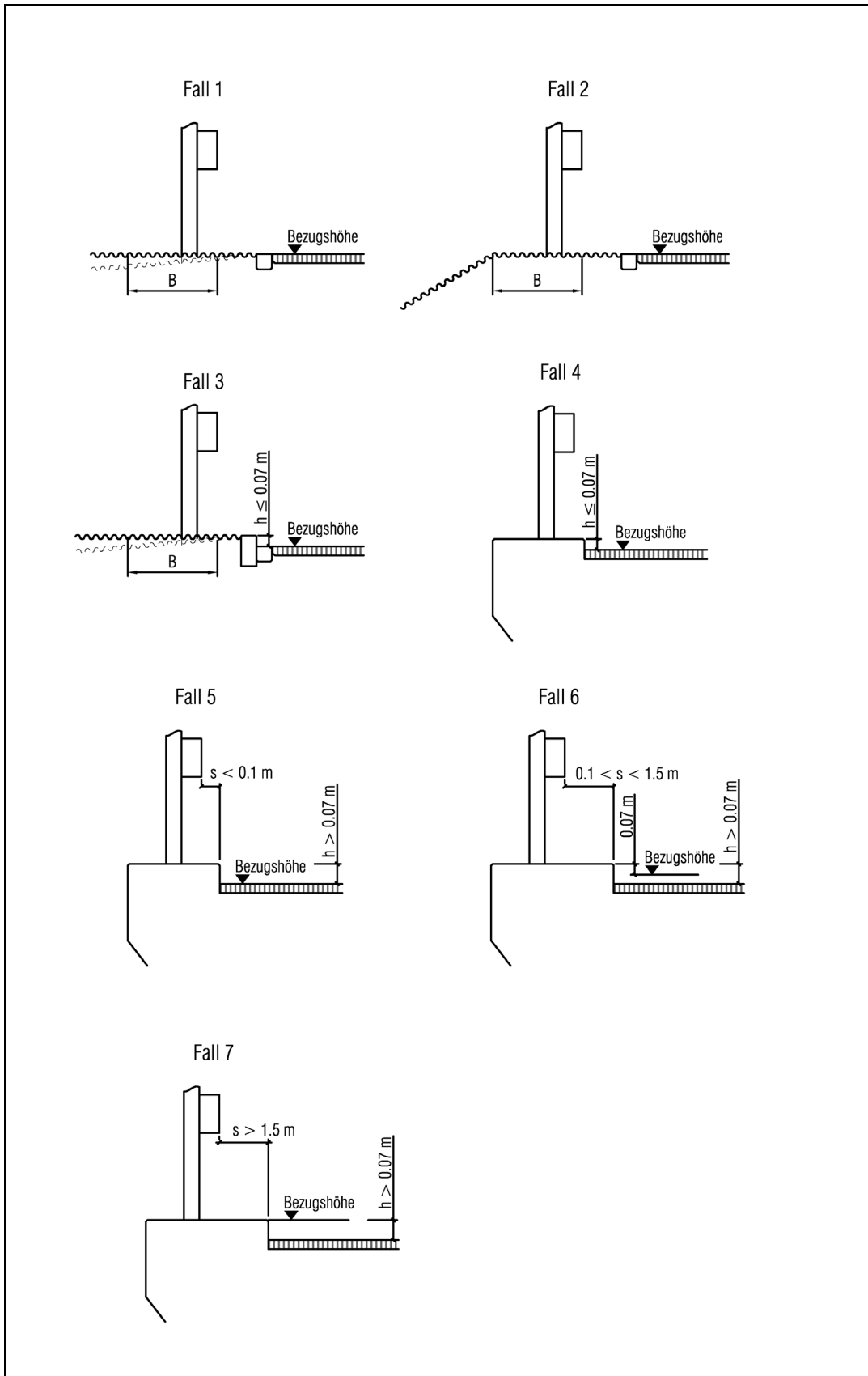
Abb. 6.1 Positionen und Bezugshöhen System 2111 (Anwendung, siehe Ziffer 6.2).
