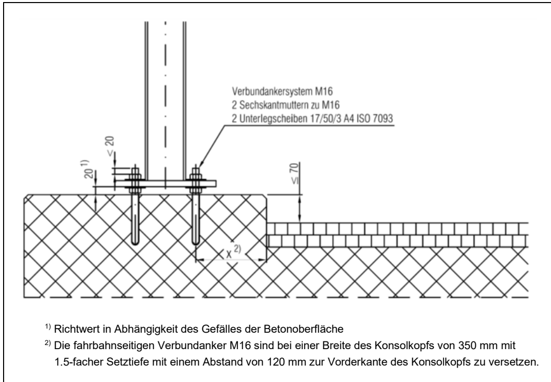
Abb. 7.2 Pfosten mit Fussplatte und Verbundanker auf Bauwerk.
