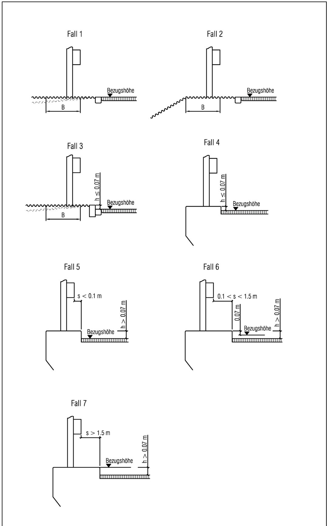
Abb. 6.1 Positionen und Bezugshöhen System 6811 (Anwendung, siehe Ziffer 6.2).
