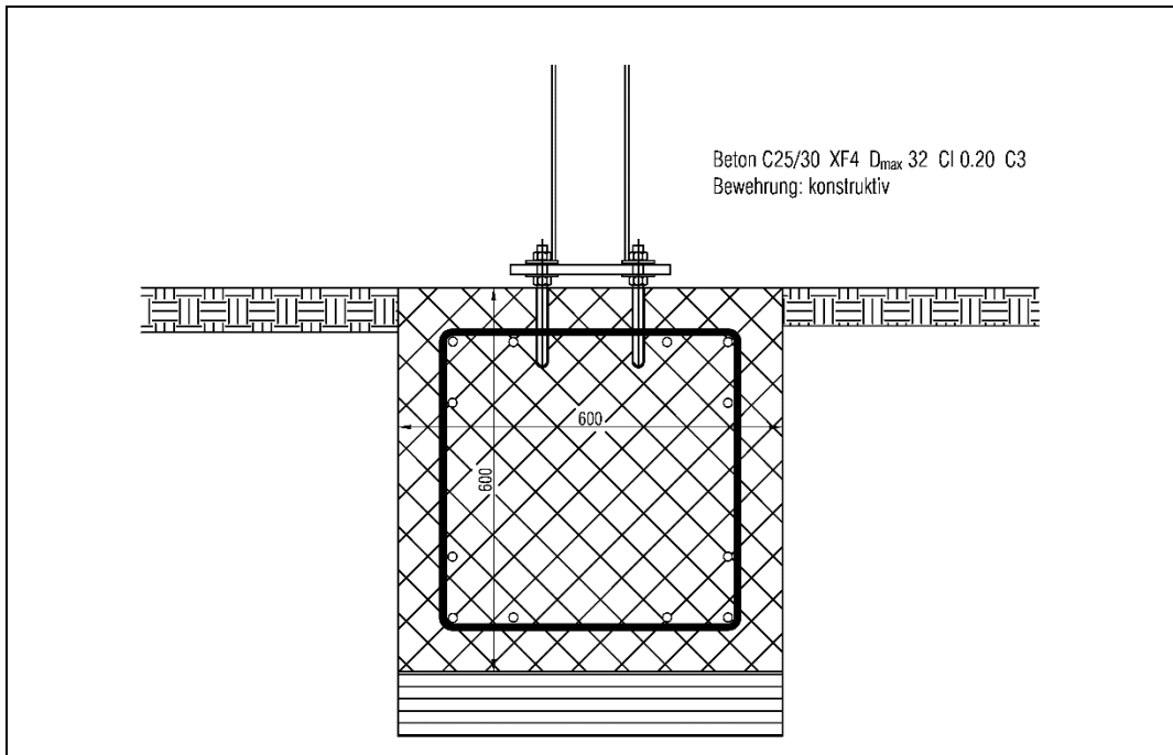
Abb. 7.3 Streifenfundament System mit Pfosten IPE 120.
