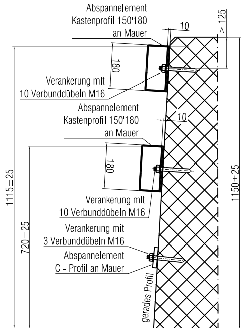
Schnitt A-A
