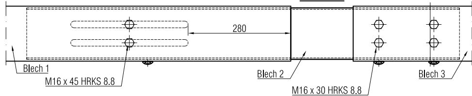
Detail D: C - Profil 50'100
