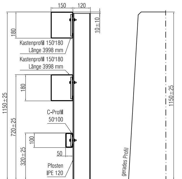
Schnitt B-B
