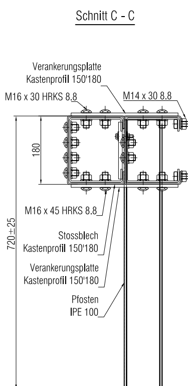
Kastenprofil 150'180 Länge 3998 mm
