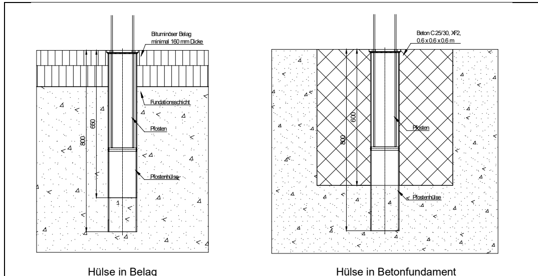
Abb. 7.1 Pfofen in Hülse.
