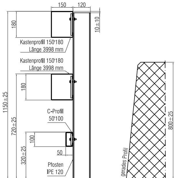
Schnitt B-B
