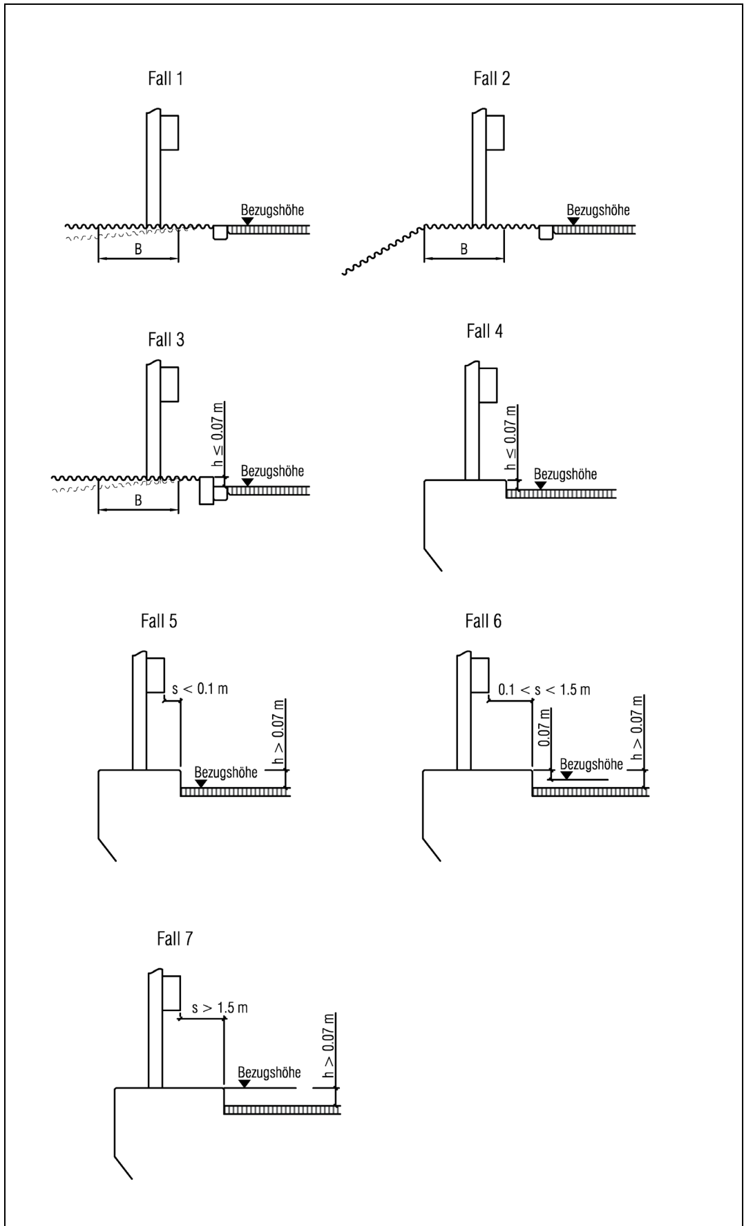
Abb. 6.1 Positionen und Bezugshöhen System 6611 (Anwendung, siehe Ziffer 6.2).
