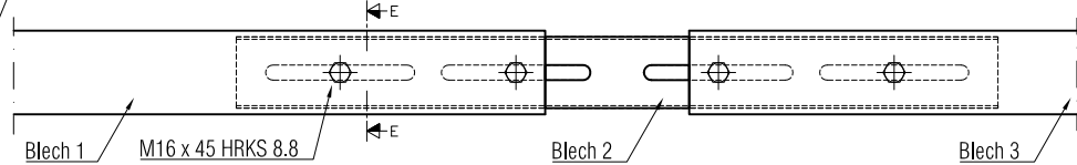
Detail D: C - Profil 50'100
