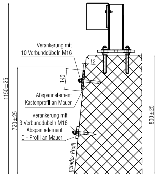
Schnitt A-A
