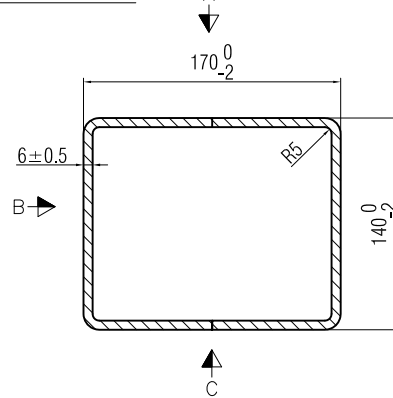
Querschnitt Blech 2
