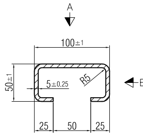
Querschnitt Blech 1 / 3
