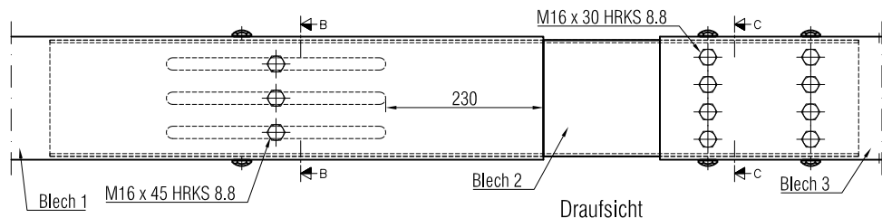
Detail A: Kastenprofil 150'180
