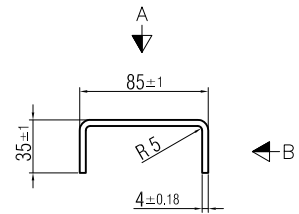
Querschnitt Blech 2
